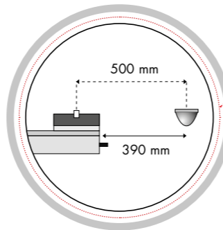
CORSA ORIZZONTALE TAMPONE Schema della corsa orizzontale del tampone in fase di stampa
